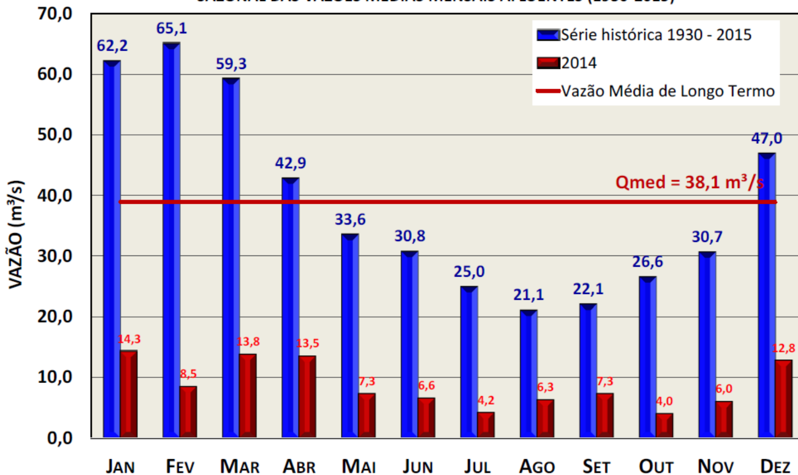
SISTEMA CANTAREIRA (ATIBAINHA, CACHOEIRA E JAGUARI/JACAREÍ) DISTRIBUIÇÃO SAZONAL DAS VAZÕES MÉDIAS MENSAIS AFLUENTES (1930-2015)
